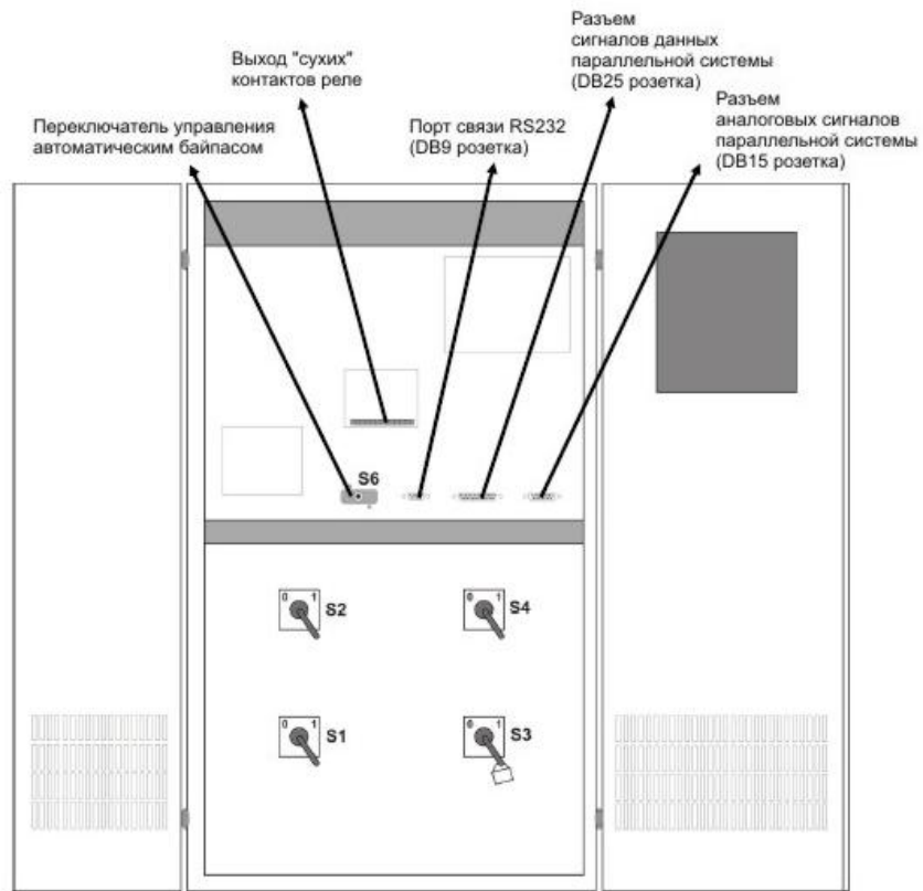
Рис. 14 Расположение переключателей и разъемов СБП 80 кВА.
