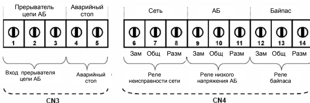
Рис.5 Назначение выводов подключения «сухих» контактов.
