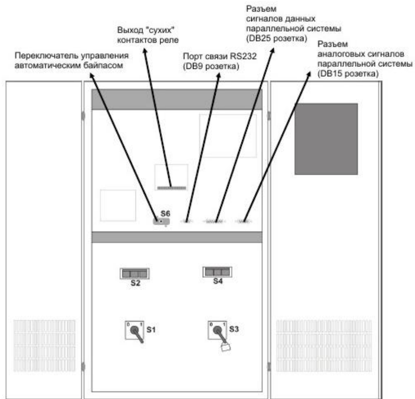
Рис. 13 Расположение переключателей и разъемов СБП 40-60 кВА.
