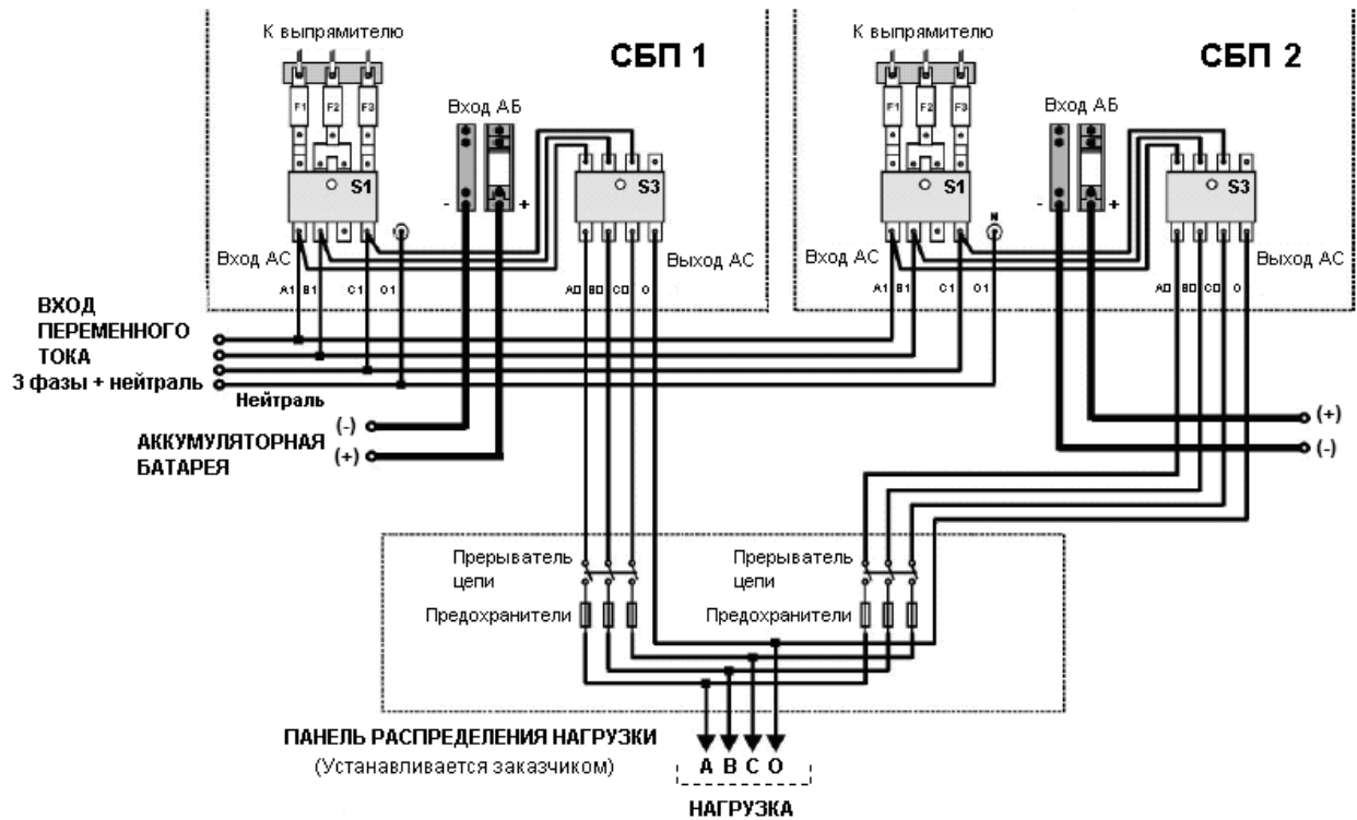
Рис. 11 Подключение сети и нагрузки при параллельной работе двух СБП 40-60-80 кВА.
