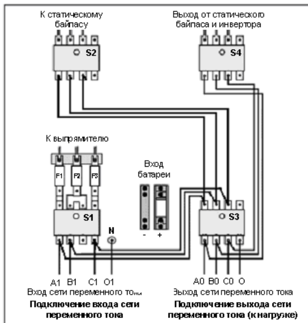
Рис. 6 Подключение кабелей СБП 40-60 кВА.
