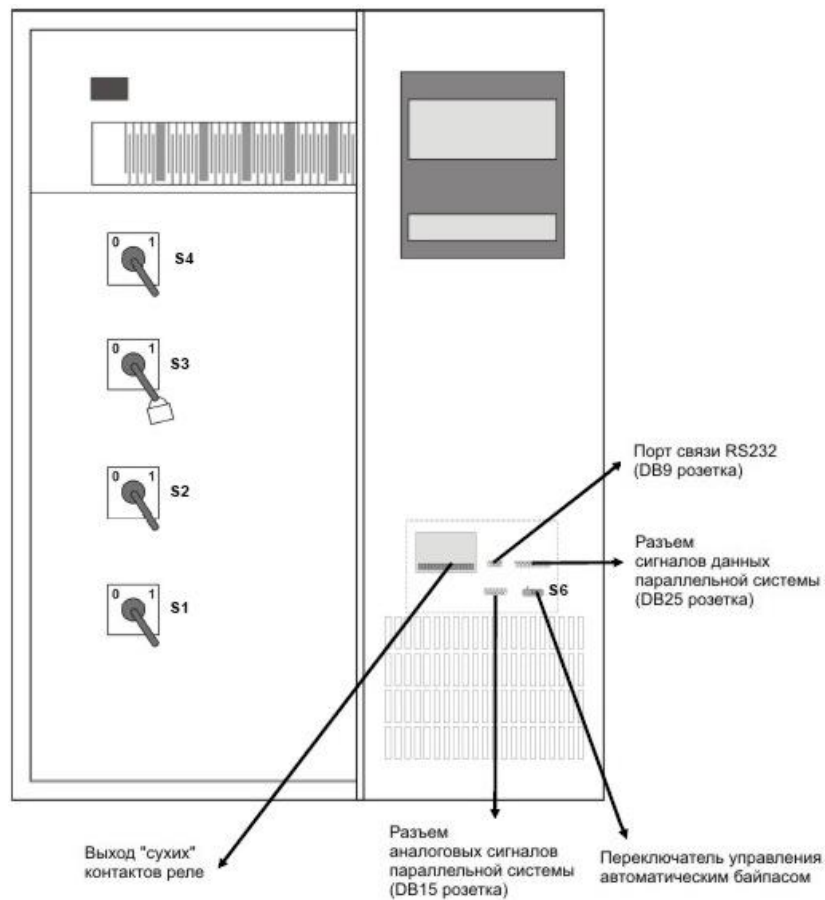
Рис. 15 Расположение переключателей и разъемов СБП 100-120-150-200 кВА.
