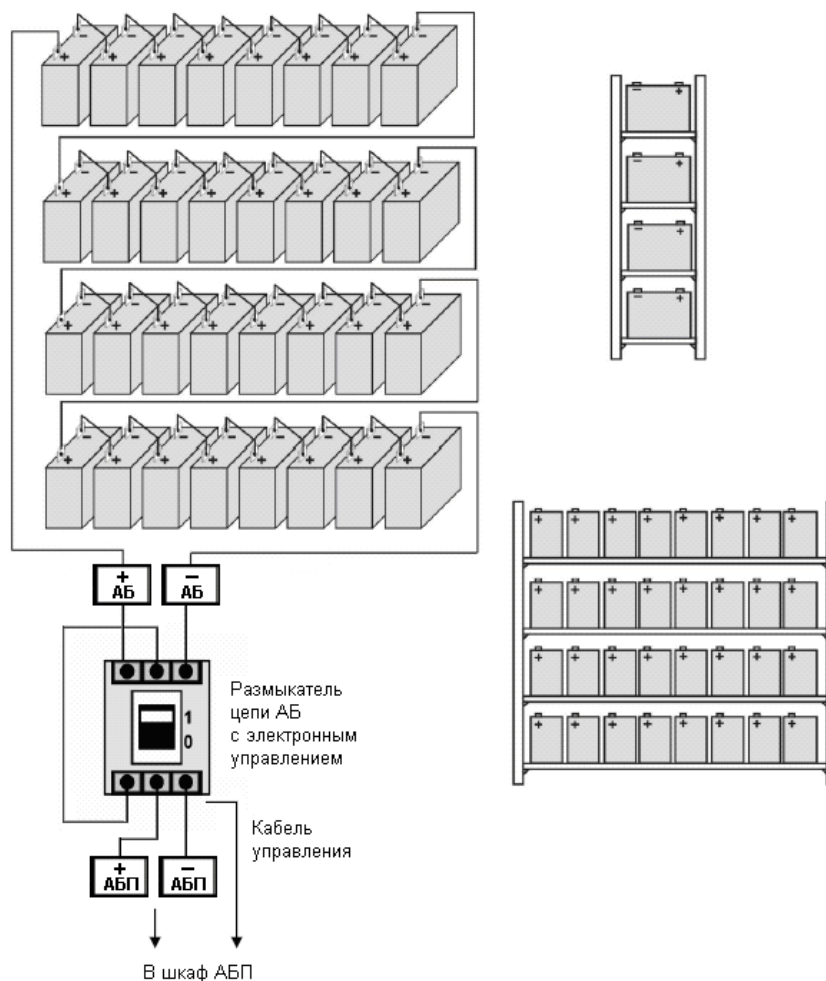
Рис. 9 Подключение аккумуляторной батареи, расположенной на стеллаже, к АБП (с использованием размыкателя цепи АБ).
