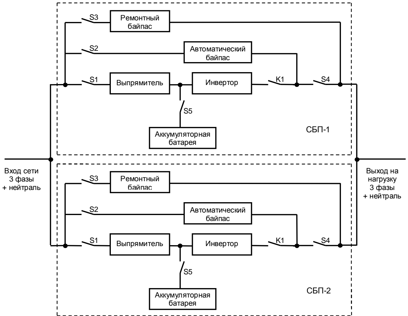
Рис.3 Структурная схема при параллельном включении двух СБП.
