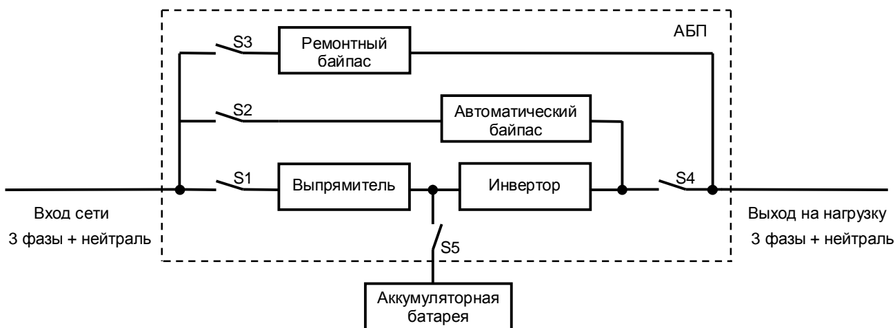
Рис. 1 Структурная схема СБП при питании выпрямителя и байпаса от одного источника.
