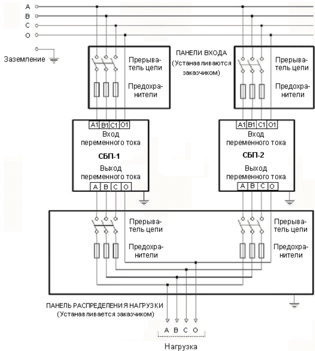
Рис. 10 Параллельное соединение двух СБП.
