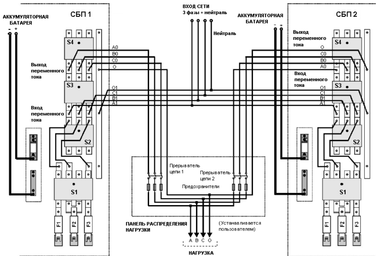
Рис. 12 Подключение сети и нагрузки при параллельной работе двух СБП 100-120-150-200 кВА.
