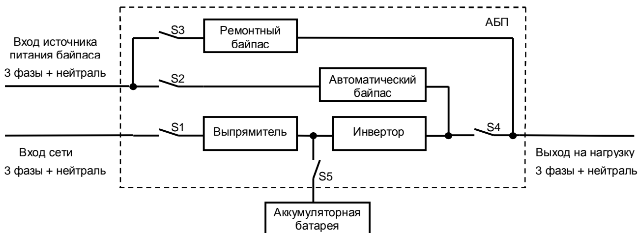
Рис. 2 Структурная схема СБП при питании байпаса от отдельного источника.
