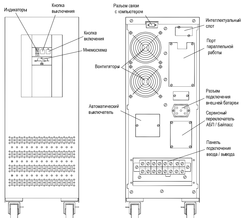
Рис. 7 Вид СБП 10 кВА спереди и сзади.
