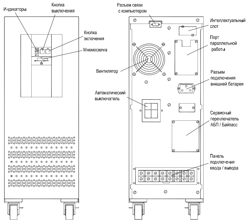
Рис. 6 Вид СБП 6 кВА спереди и сзади.
