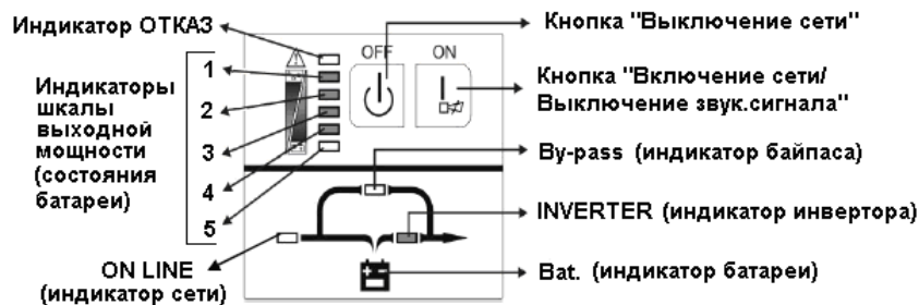
Рис. 2 Панель управления и индикации.
