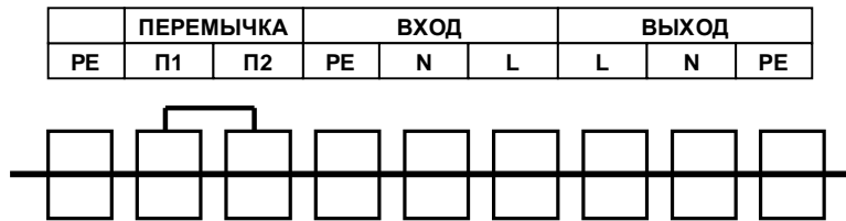
Рис 5. Схема подключения СБП на мощность 10 кВА.
