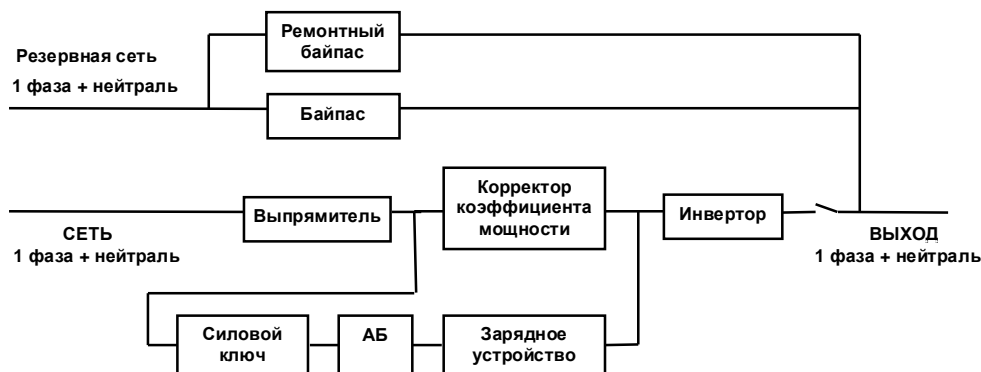
Рис. 1 Структурная схема СБП при использовании в качестве резервной сети отдельного источника питания.
