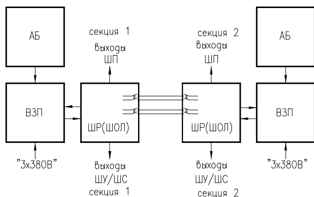
Структурная схема. Вариант 2.5
