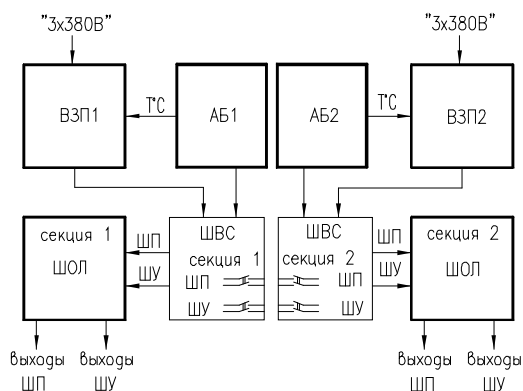
Структурная схема. Вариант 2.4
